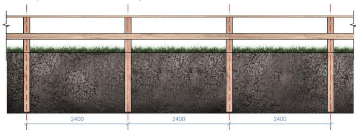
Ограждение ОГ-1 на деревянных столбах
