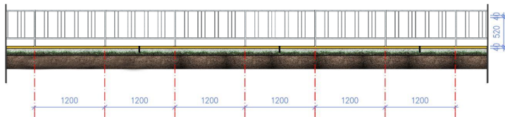
Ограждение ОГ-3 на бетонном основании (Бордюр дорожный)
