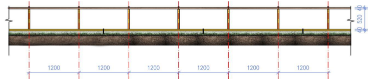
Ограждение ОГ-2 на бетонном основании (Бордюр дорожный)
